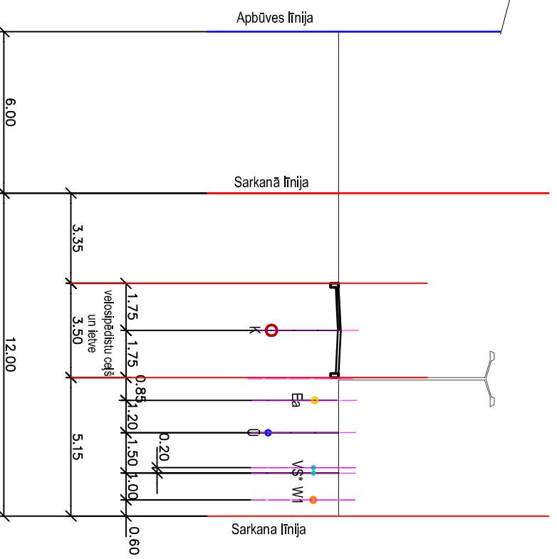
Šķēršprofils 3-3 Peldu iela
