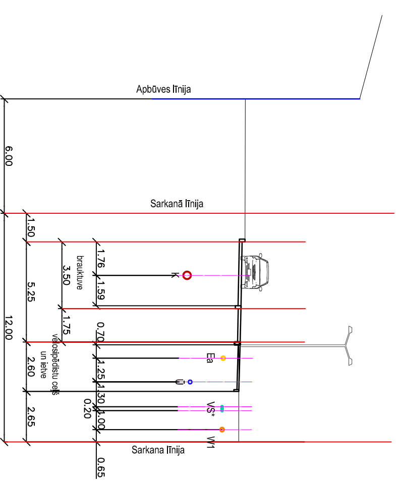
Šķēršprofils 2-2 Peldu iela
