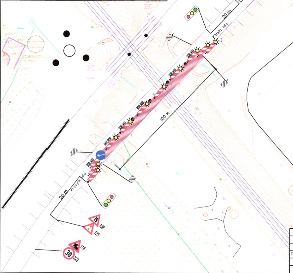
Pagaidu ceļa zīmju shēma, Kraujas iela, Daugavpilī.
