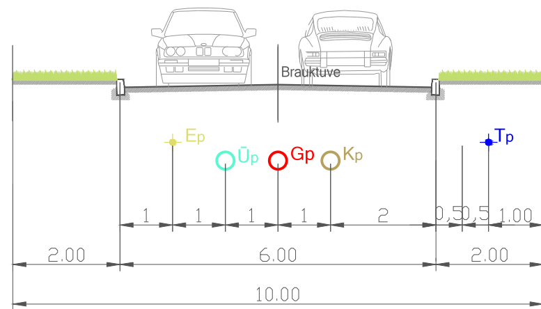
Iebrauktuves šķēršprofils 1-1
